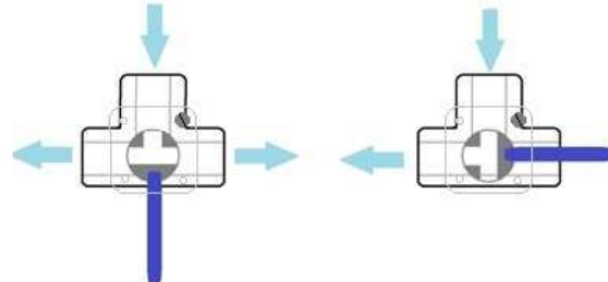
Sfera a "T" deviatrice
