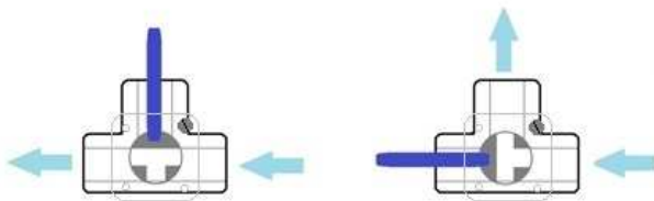
Sfera a "T" deviatrice
